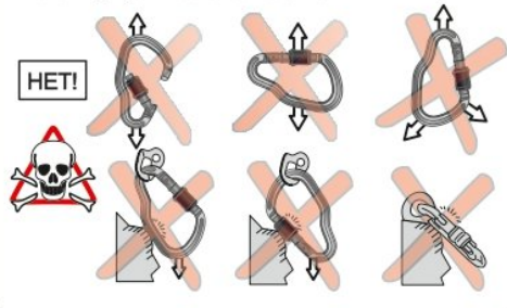
Рис. 5. Недопустимое использование
