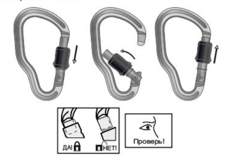
Рис. 3. Открытие / закрытие / фиксация запорного элемента
