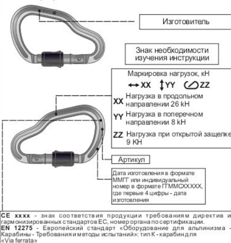
Рис. 2. Маркировка изделий
