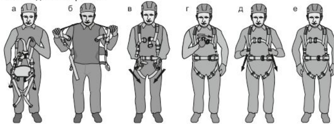
Рис. 4. Надевание привязи
