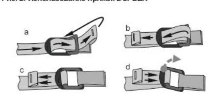
Рис. 2. Использование пряжек DUPLEX
