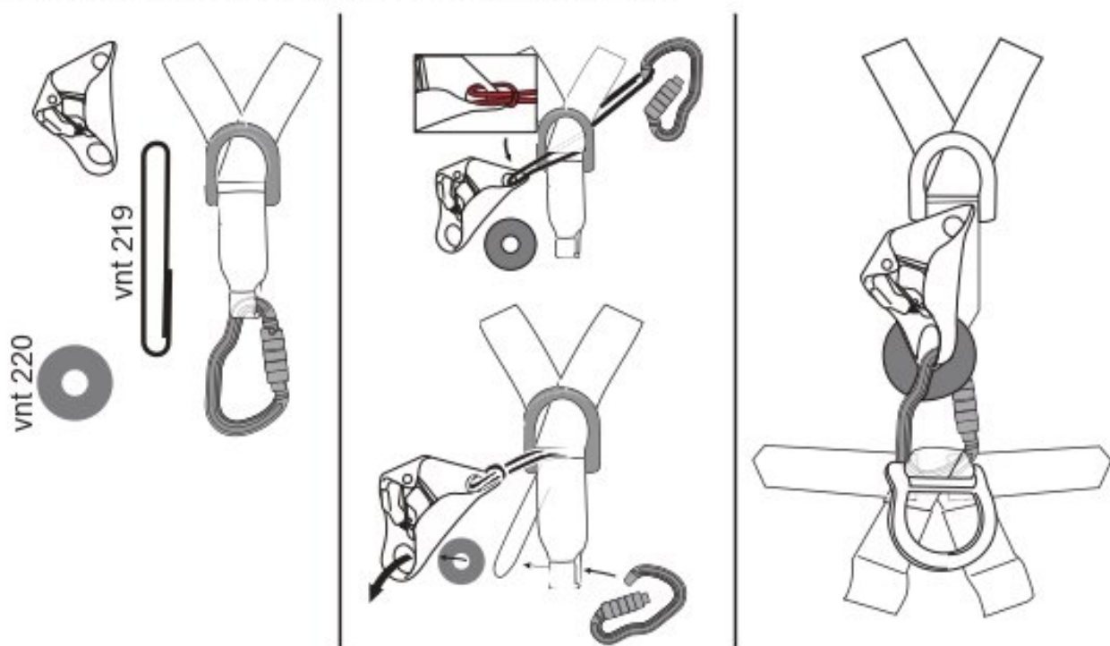
Рис. 15. Способ интеграции зажима «Кроль»
