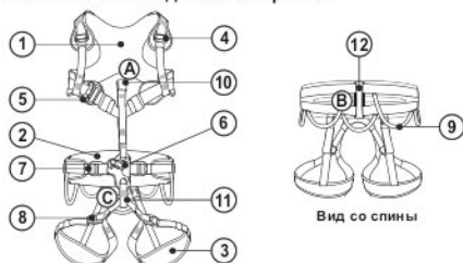
Рис. 1. Внешний вид и состав привязи
