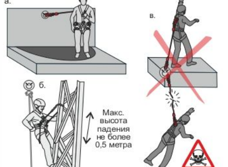
Рис. 11. Использование стропов без амортизатора
