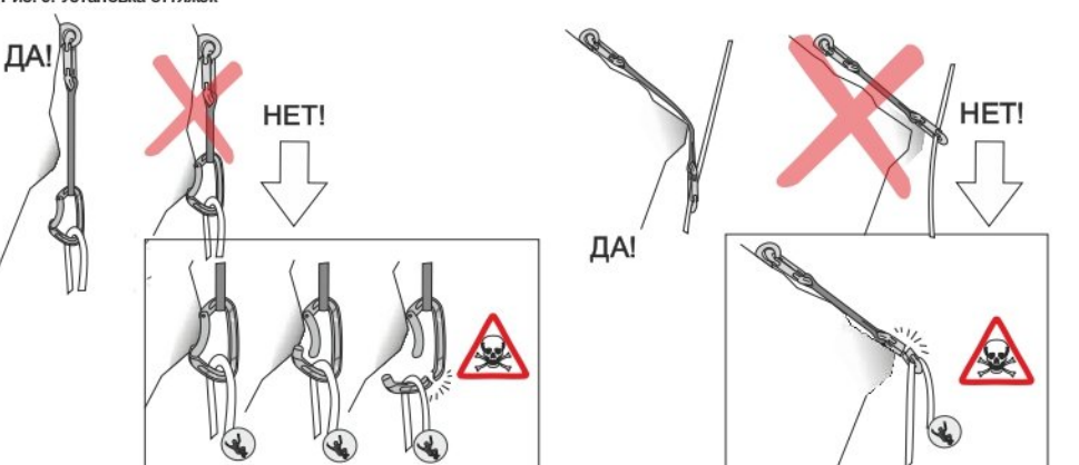
Рис. 6. Установка оттяжек
