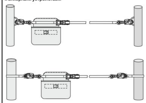
Рис. 4. Способы присоединения к анкерным устройствам
