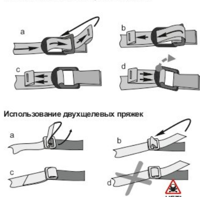
Рис. 2. Использование пряжек DUPLEX
