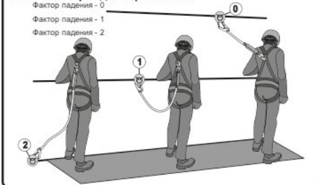
Рис. 11. Использование стропов без амортизатора
