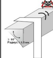
Рис. 5. Недопустимые параметры опоры
