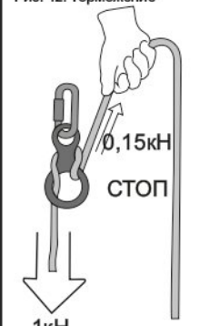
Рис. 12. Торможение
