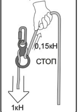
Рис. 12. Торможение
