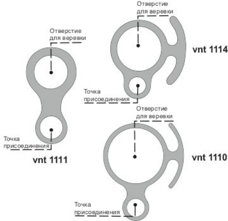
Рис. 2. Маркировка изделия
