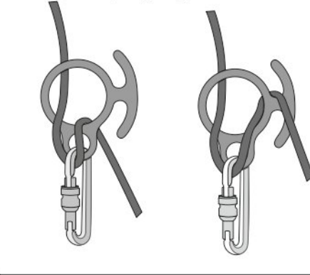
Рис. 8. Организация системы для спуска
