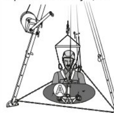
Рис. 17. Пример организации системы канатного доступа
