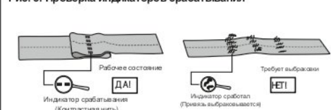
Рис. 5. Проверка индикаторов срабатывания
