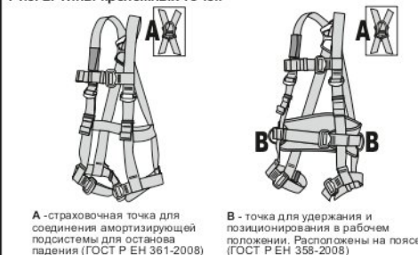
Рис. 2. Типы крепежных точек
