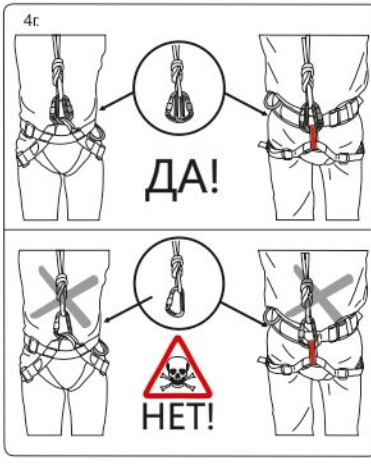
Рис. 7. Использование грудных обвязок
