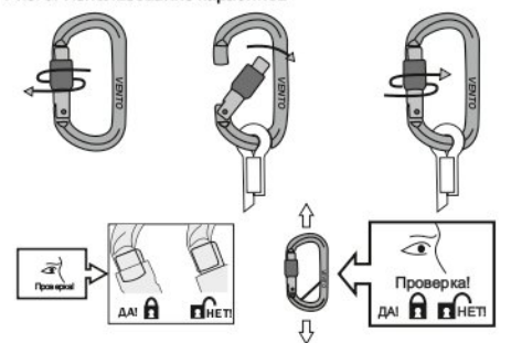
Рис. 3. Использование карабинов
