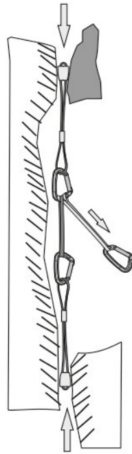
Рис. 7. Извлечение закладки
