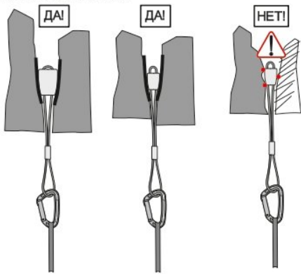
Рис. 4. Установка закладки
