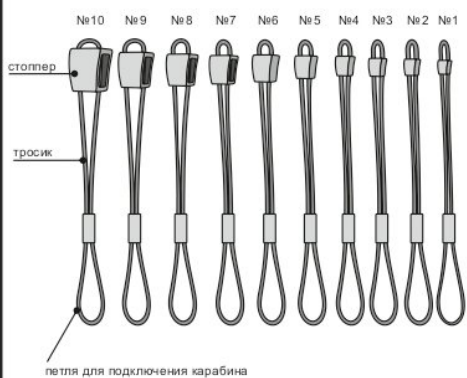
Рис. 2. Маркировка
