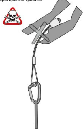
Рис. 5. Перетирание тросика
