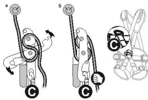
Рис. 6. Функционирование устройства
