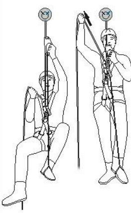
Рис. 13. Подъем с использованием зажима со стременом
