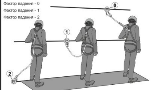
Рис. 8. Графическая схема к определению фактора падения
