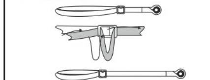
Рис. 7. Регулировка длины
