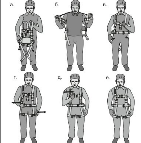
Рис. 5. Способы надевания привязи
