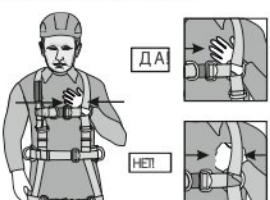
Рис. 11. Способ организации удерживающей системы
