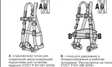
Рис. 2. Типы крепежных точек
