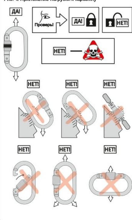
Рис. 4. Приложение нагрузки к карабину
