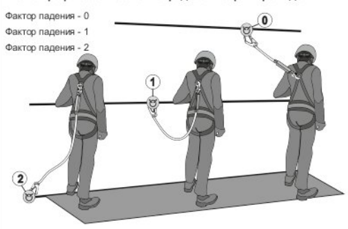
Рис. 8. Графическая схема к определению фактора падения
