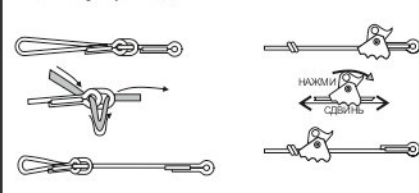
Рис. 7. Регулировка длины
