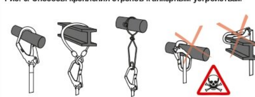
Рис. 6. Способы крепления стропов к анкерным устройствам
