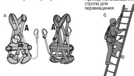
Рис. 4. В страховочных системах допускается использование только стропы с амортизатором рывка
