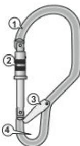
Рис. 1. Общий вид и составные детали соединительных элементов
