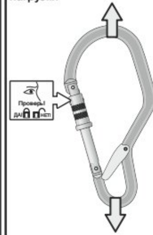
Рис. 4. Приложение нагрузки
