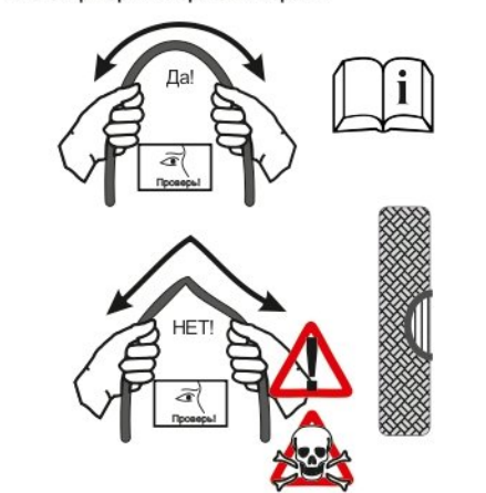
Рис. 3. Критерии выбраковки веревок
