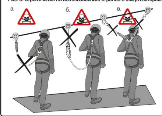
Рис. 8. Ограничения по использованию стропов с амортизатором
