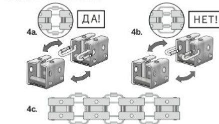
Рис. 4. Сборка комплекта
