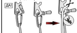
Рис. 11. Проверка изделия
