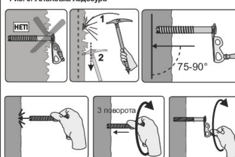
Рис. 6. Установка ледобура
