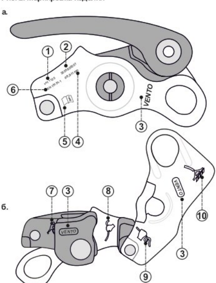
Рис. 2. Маркировка изделия
