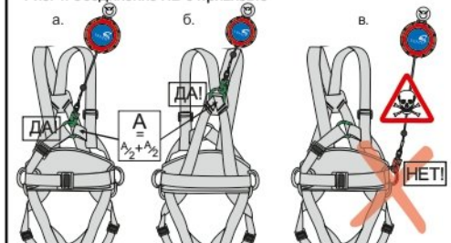
Рис. 4. Соединение НВ с привязью
