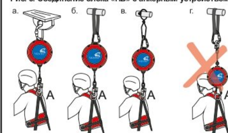
Рис. 3. Соединение блока «НВ» с анкерным устройством
