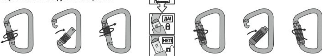
Рис. 4. Открытие / закрытие / фиксация запорного элемента с ручным запирающим
