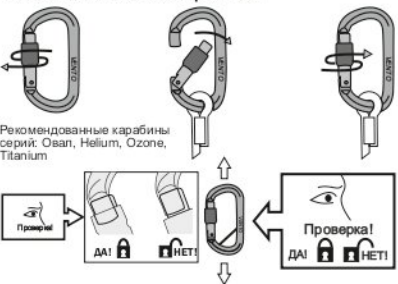
Рис. 5. Использование карабинов
