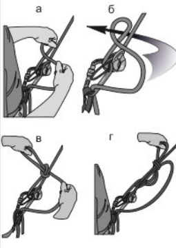
Рис. 12. Страховка 2 человек
