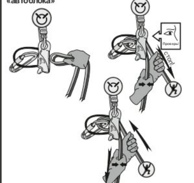
Рис. 13. Запрещенные способы
