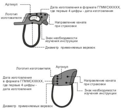
Рис. 2. Маркировка изделия
