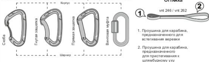
Рис. 1. Составные части и типы запирающих элементов
