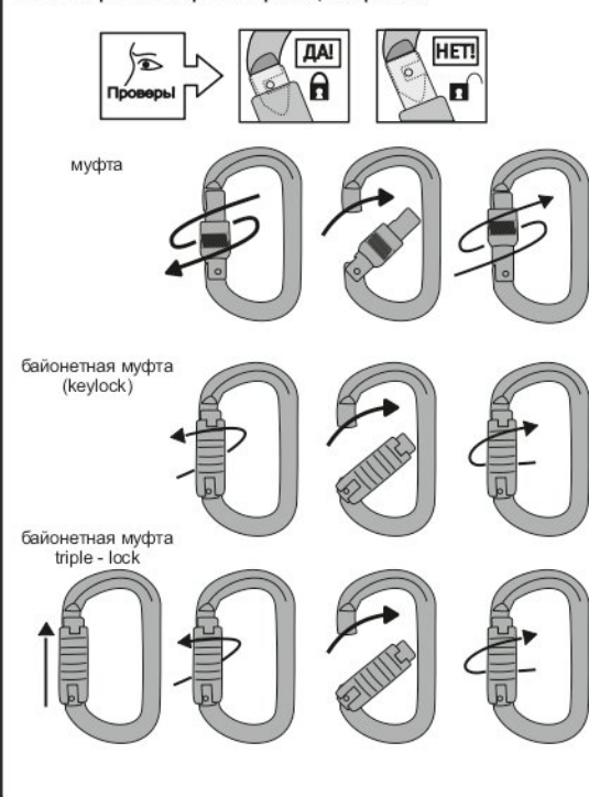
Рис. 3. Открытие / закрытие / фиксация карабина
