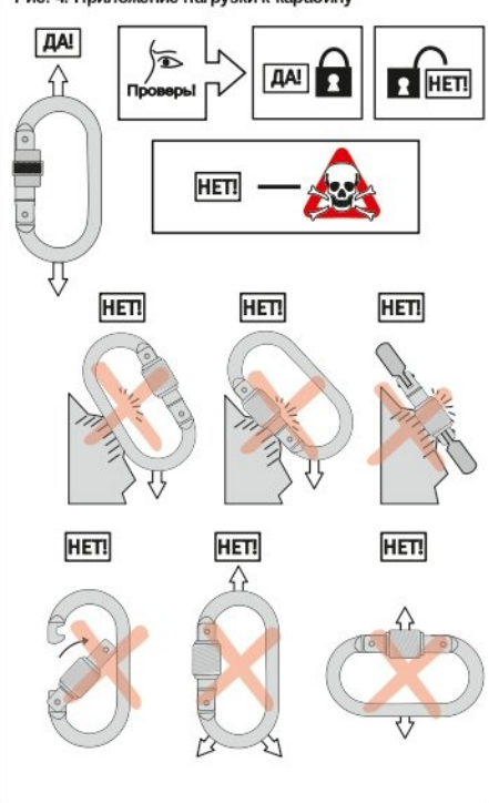
Рис. 4. Приложение нагрузки к карабину
