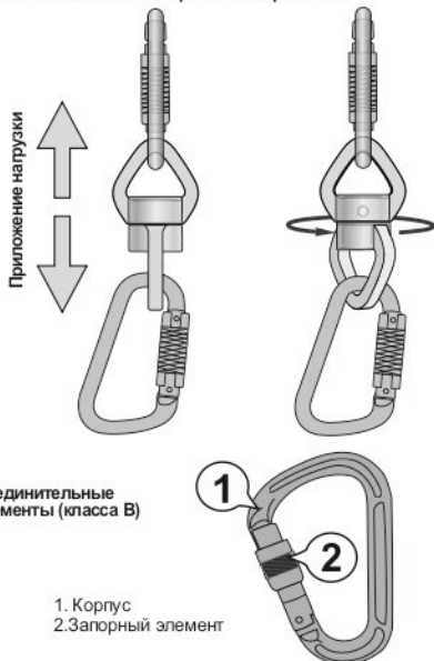
Рис. 2. Использование вертлюга с карабинами
