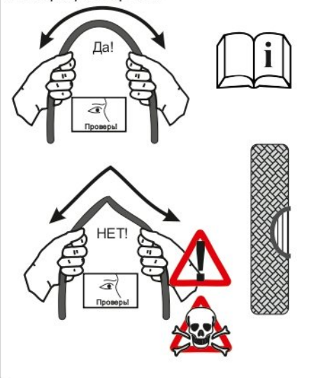
Рис. 3. Критерии выбраковки
