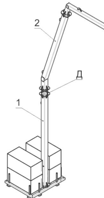
Рисунок 3 - Схема сборки стойки 1 - Стойка низ, 2 -Стойка верх.
