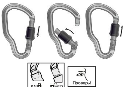
Рис. 3. Открытие / закрытие / фиксация запорного элемента
