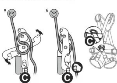
Рис. 3б. Эвакуация
