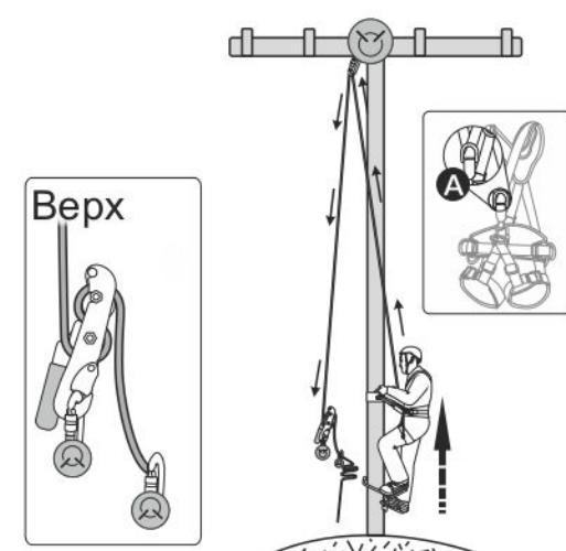
Рис. 4а. Предустановленная система, подъем
