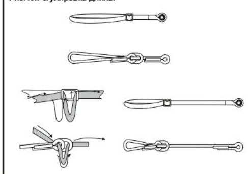
Рис. 10. Регулировка длины
