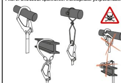
Рис. 5. Способы крепления к анкерным устройствам
