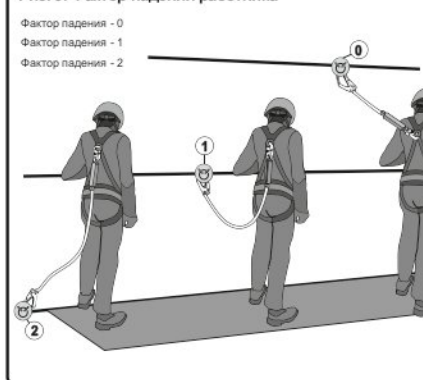
Рис. 11. Использование стропов без амортизатора
