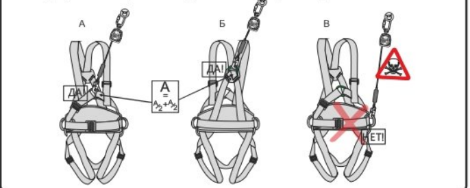
Рис. 4. Допустимые варианты соединения «НВ-02 трос» с привязью
