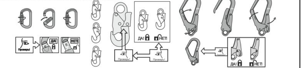
Рис. 6. Ограничения по способу приложения нагрузки (относятся ко всем типам карабинов) См. Инструкцию по применению карабинов
