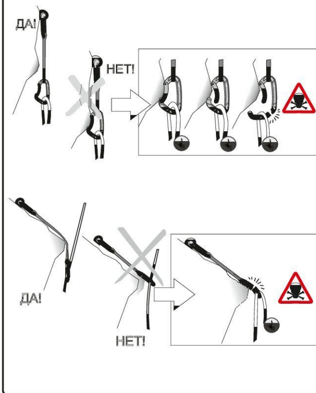
Рис. 4. Установка оттяжек
