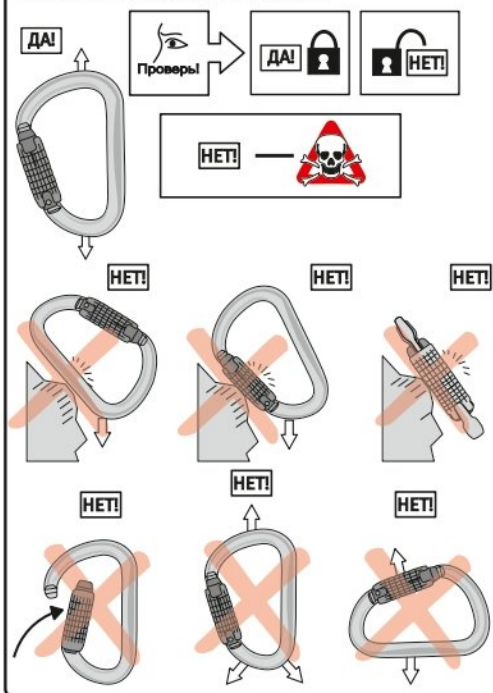
Рис. 4. Приложение нагрузки к карабину
