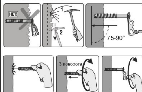
Рис. 6. Установка ледобура
