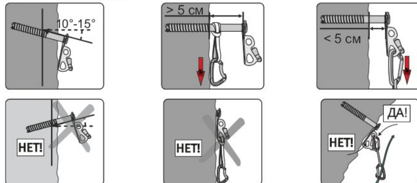
Рис. 8. Предостережение
