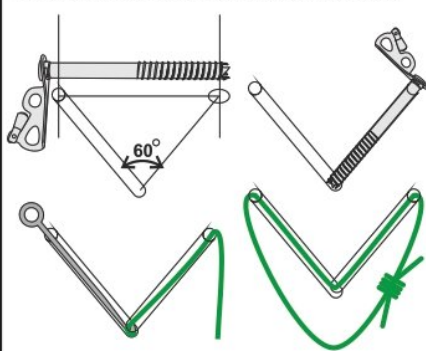
Рис. 7. Положение анкерного устройства
