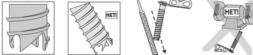
Рис. 12. Заточка коронки
