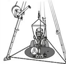
Рис. 20. Способ интеграции рабочего сиденья
