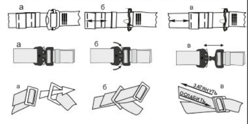
Рис. 7. Типы используемых пряжек, способы заправки
