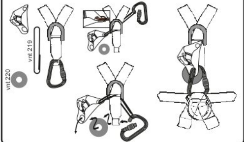
Рис. 13. Соединительно-амортизирующая подсистема
