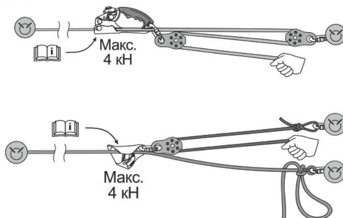
Рис. 4. Наведение переправы
