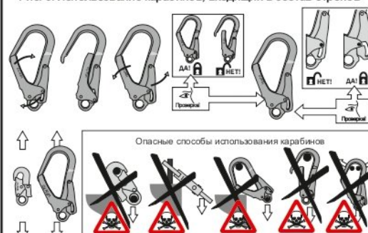
Рис. 6. Использование карабинов, входящих в состав стропов
