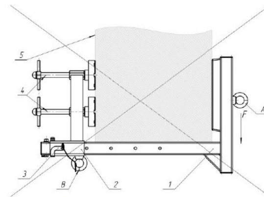
Рис. 4. 1 – врга B004-100 СБ Каркас; 2 – врга B004-200 СБ Обойма; 3 – врга B004-300 СБ Фиксатор; 4 – врга B004-202 СБ Прижим; 5 – Паралет.
