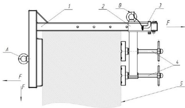
Рис. 3. Монтаж анкерного устройства. 1 – врга B004-100 СБ Каркас; 2 – врга B004-200 СБ Обойма; 3 – врга B004-300 СБ Фиксатор; 4 – врга B004-202 СБ Прижим; 5 – Паралет.
